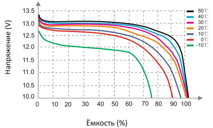
Зависимость разряда от температуры (0,5C)
