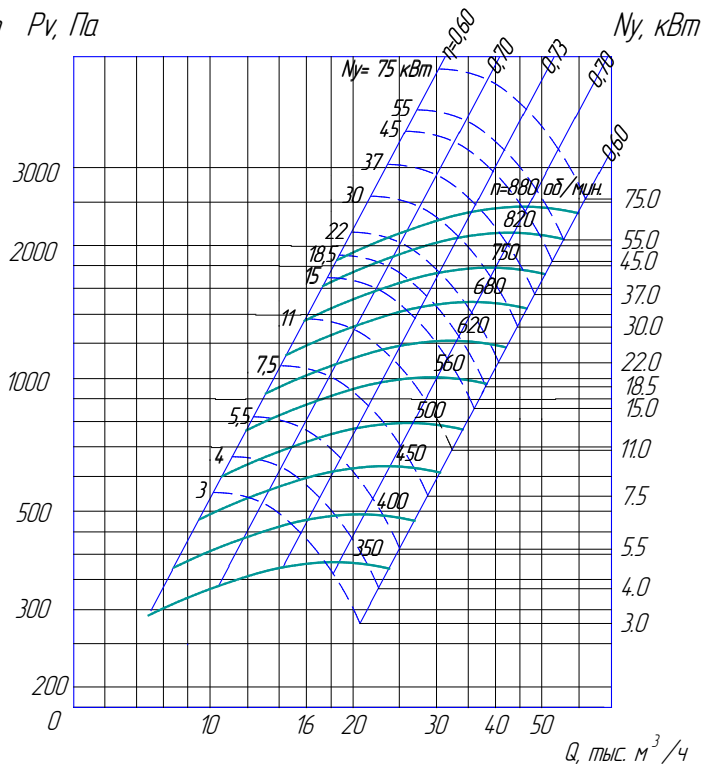
ВР 280-46-8 исп. 5
