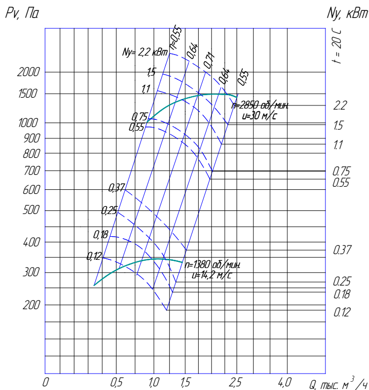
ВР 280-46-2
