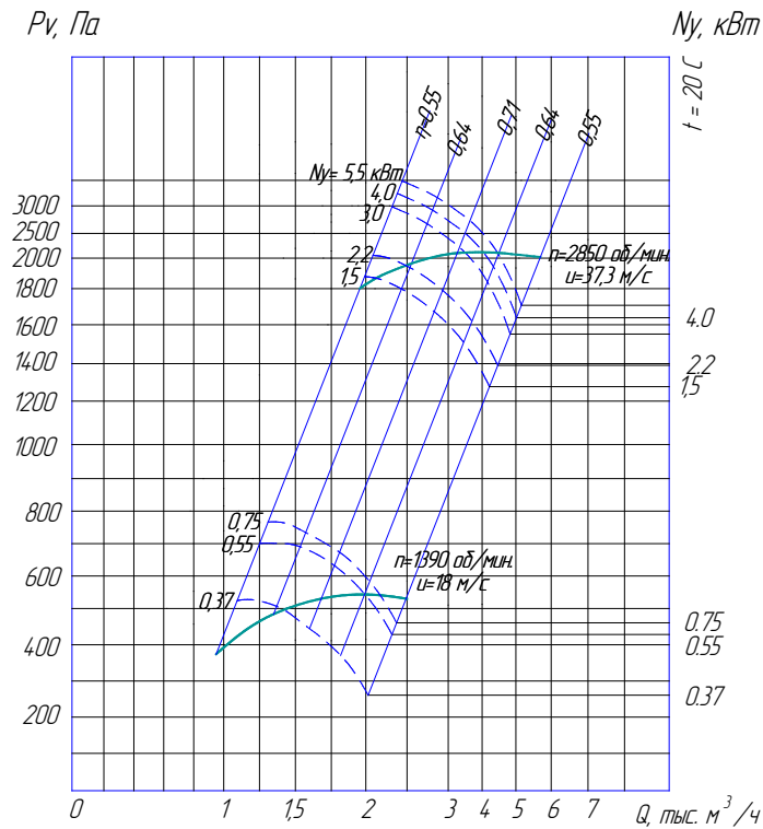
ВР 280-46-2,5
