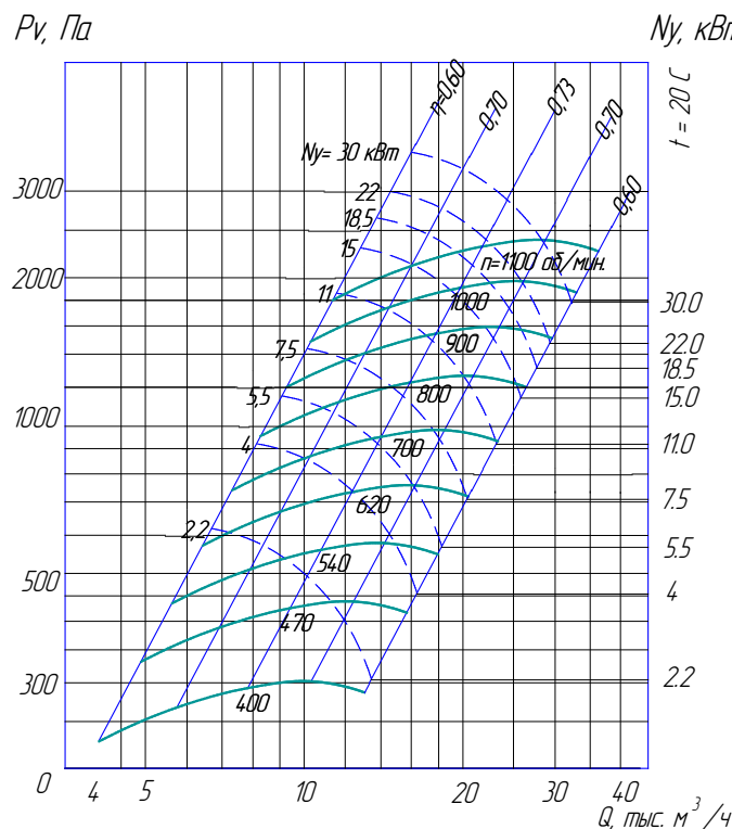
ВР 280-46-6.3 исп. 5
