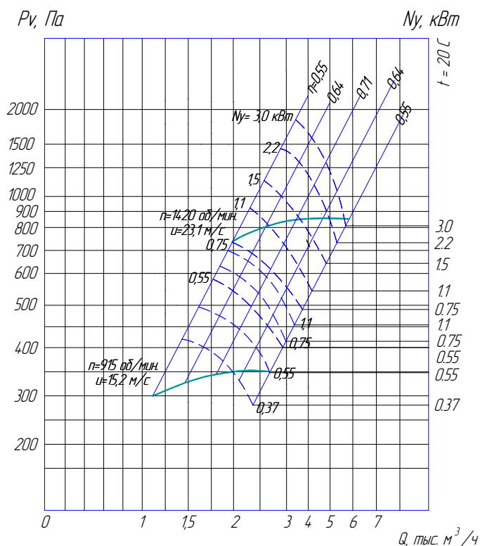
ВР 280-46-3,15
