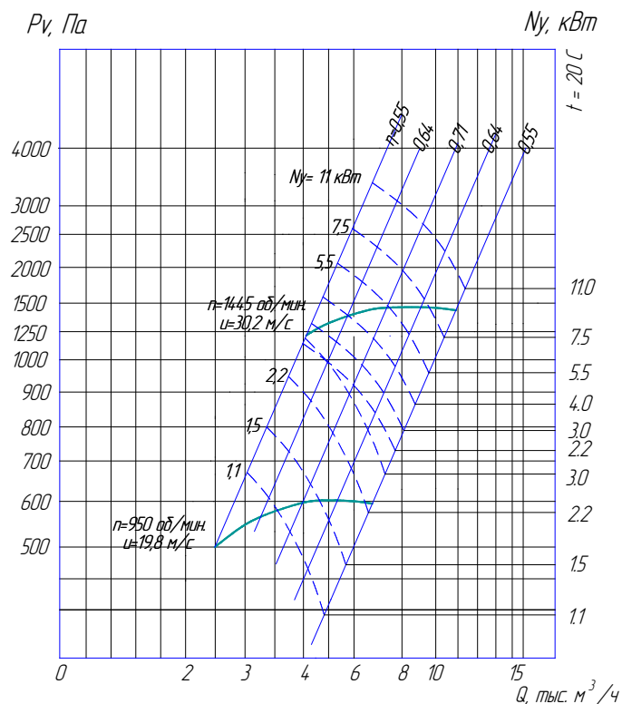
ВР 280-46-4
