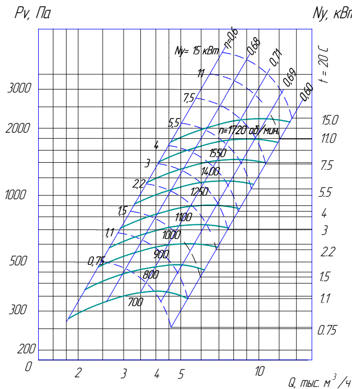
ВР 280-46-4 исп. 5
