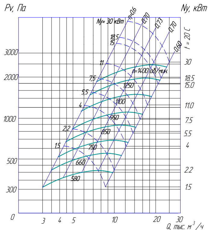
ВР 280-46-5 исп. 5
