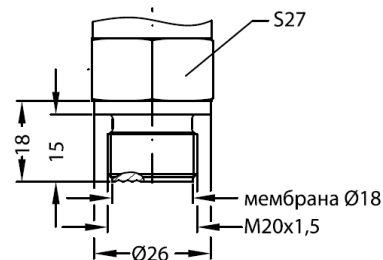
Код Z04 (M20x1.5 DIN 3852, торцевая мембрана)
