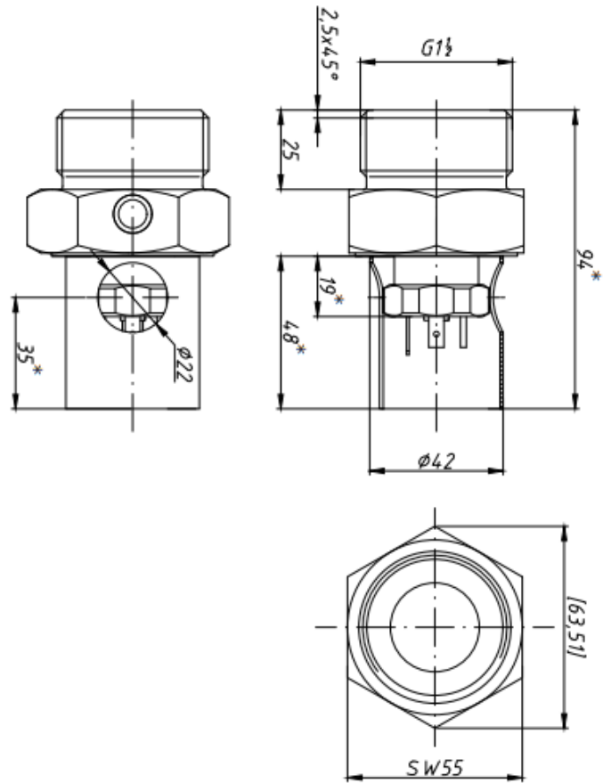
Код T33 (G1 1/2" DIN 3852, поршневая мембрана для абразивных сред)
