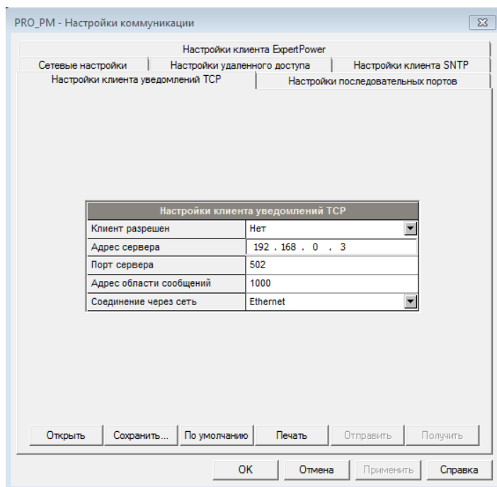
Рисунок 76 – Настройки TCP-клиента уведомлений
