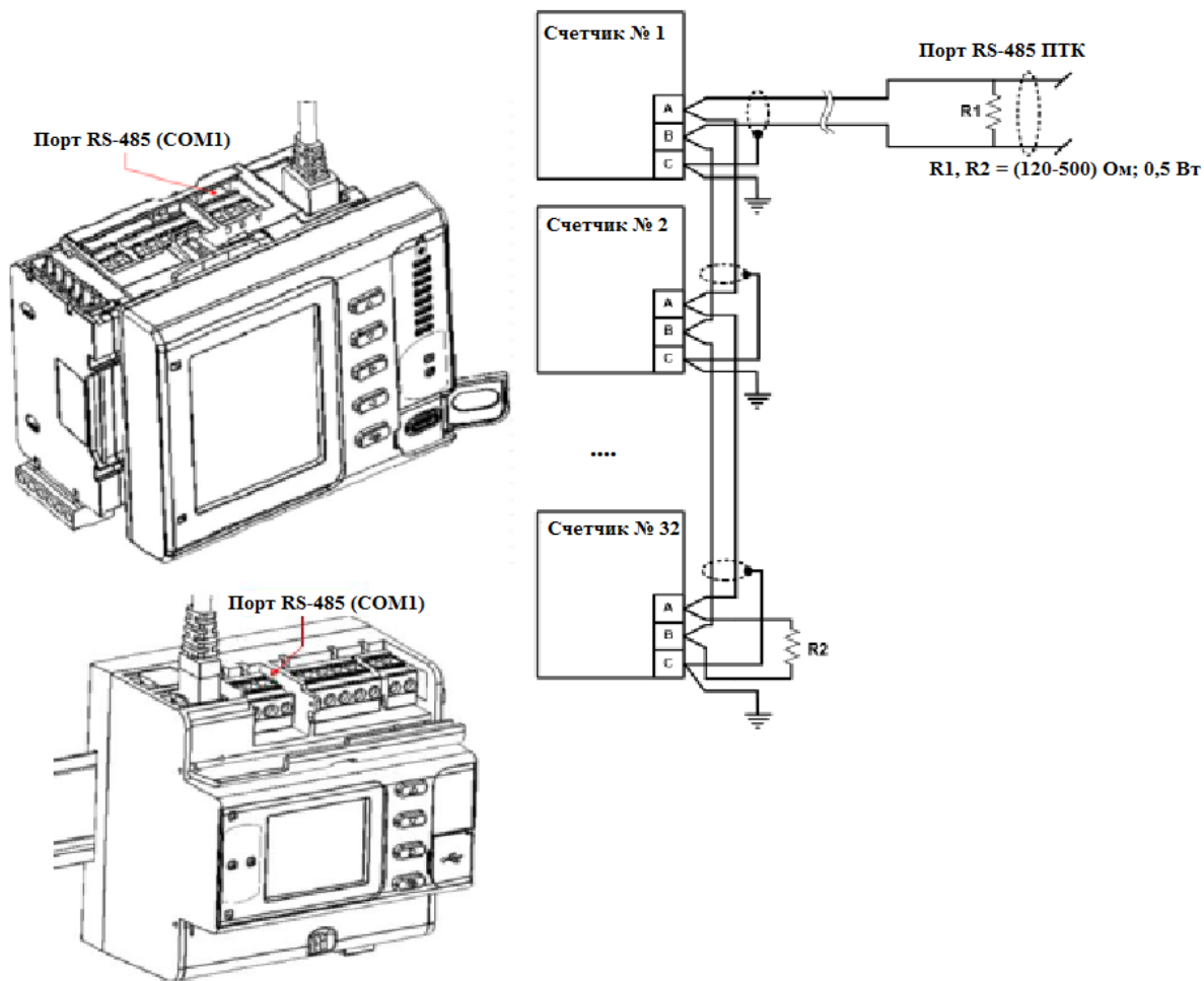
Рисунок 31 – Схема подключения порта встроенного порта RS-485 (COM1)
