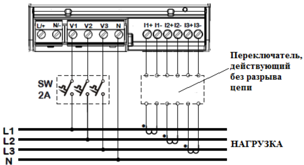
Рисунок 19 – Четырехпроводное трёхэлементное соединение звездой с использованием 3 ТТ и нейтрального провода (код настройки 4LN3)
