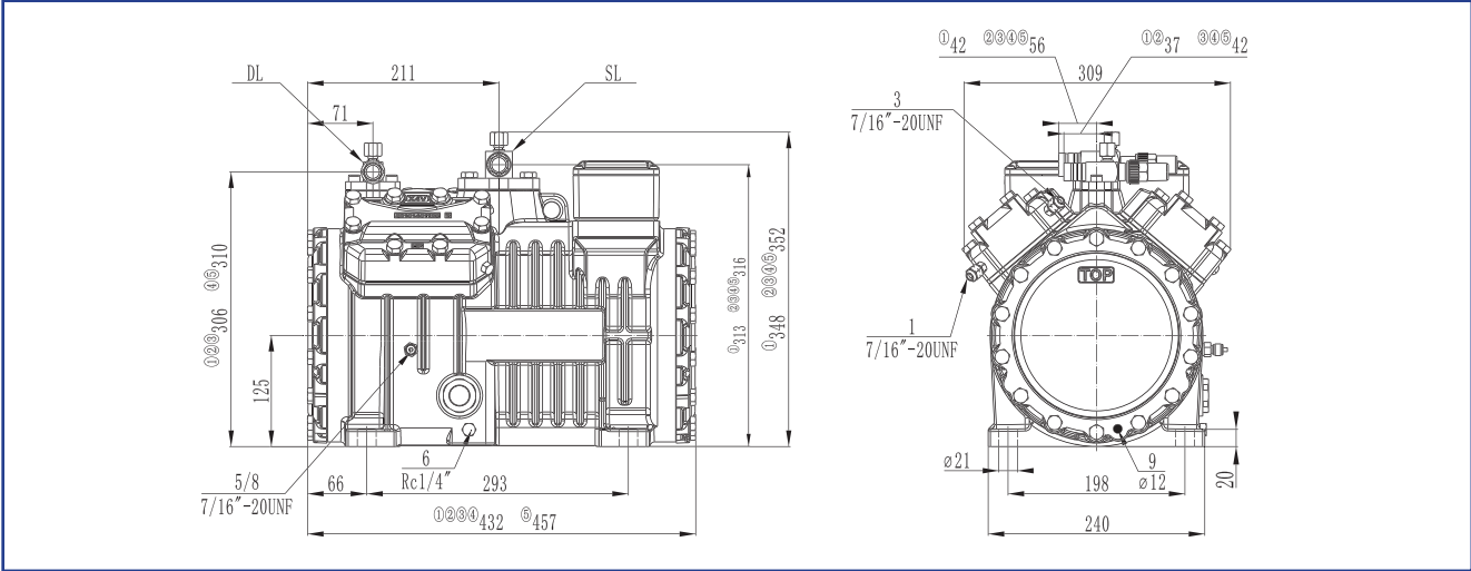
Размер соединения всасывающего и нагнетательного вентилей
