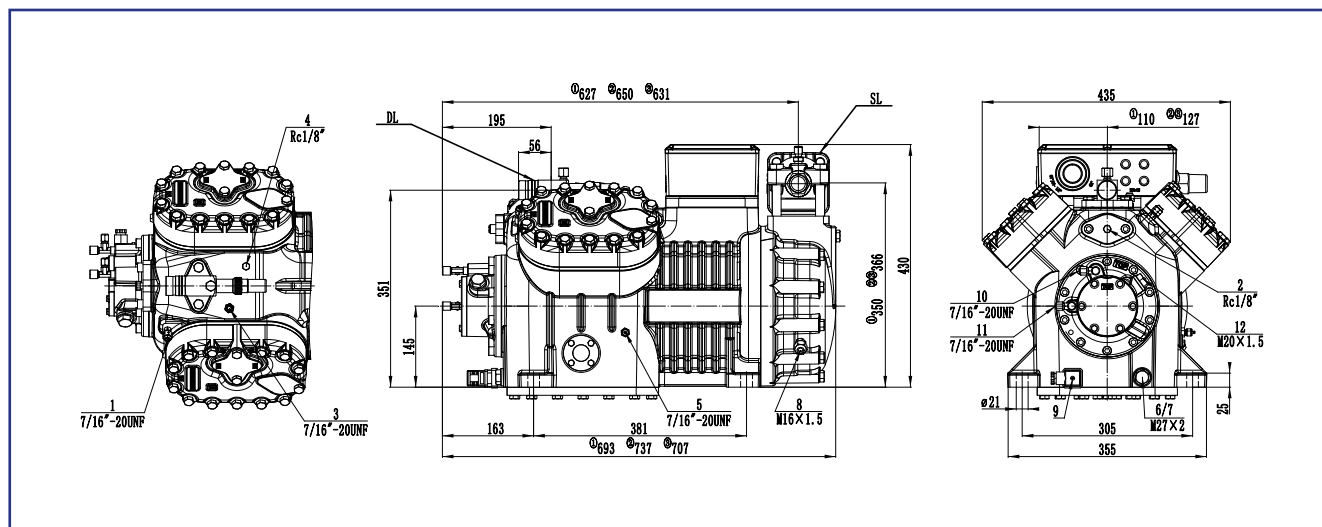
Размер соединения всасывающего и нагнетательного вентиляй
