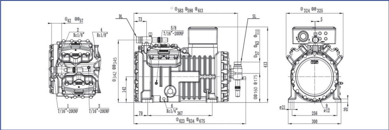
Размер соединения всасывающего и нагнетательного вентилей
