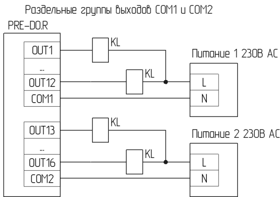
Рис. П1.1 Внешний вид и схема подключения модулей серии PRE-16DO.R-RS24
