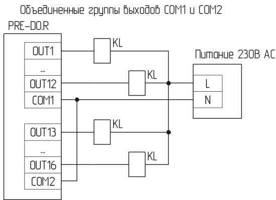
Рис. П1.1 Внешний вид и схема подключения модулей серии PRE-16DO.R-RS24
