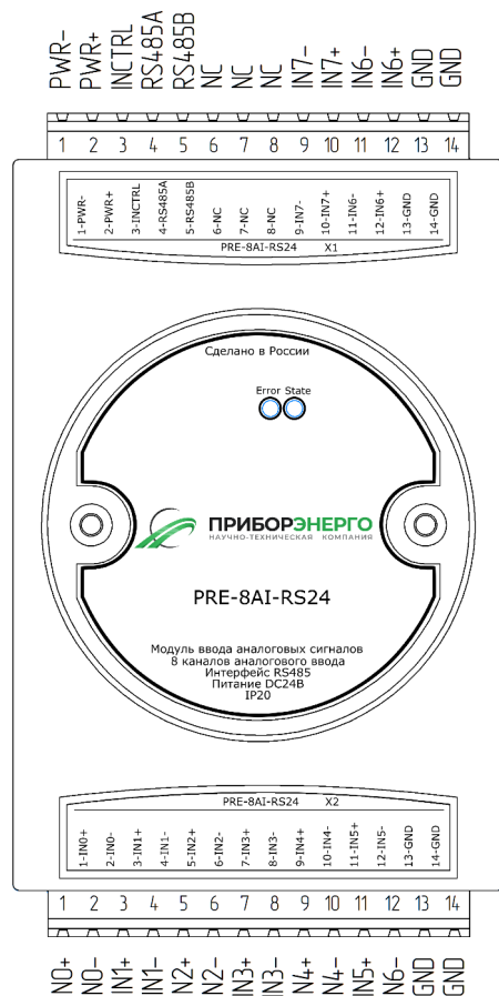
Рис. 2.1. Внешний вид и схема подключения модулей серии PRE-8AI-RS24
