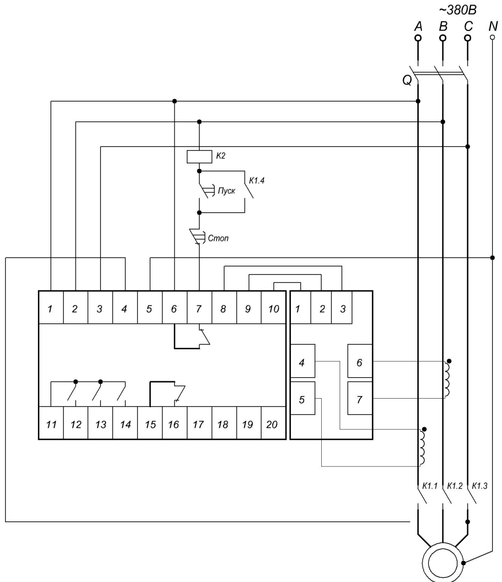
Рисунок Г.3 Схема подключения устройства защиты УЗД-3-XXXX УЗ
