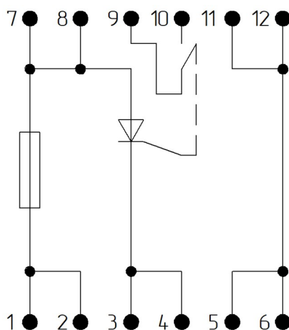
Рис.2 Схема подключения.
