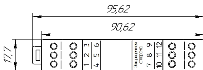
Установочные размеры Исполнение 1 сверху Исполнение 2 снизу
