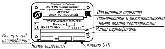
Пример таблички агрегата
