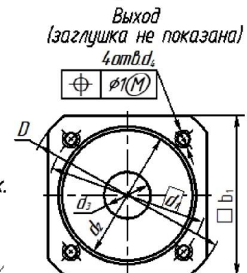
Рисунок Б.6
