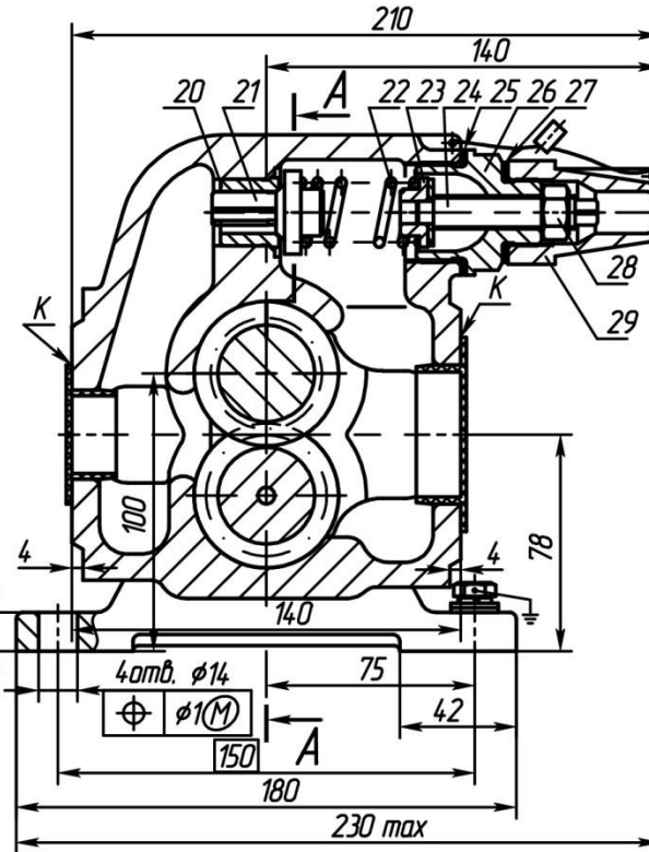
Рисунок А.2 (остальное см. рисунок А.1) Размеры в мм
