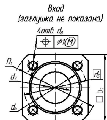
Рисунок Б.5
