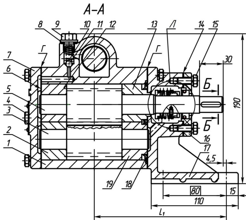
Рисунок А.1
