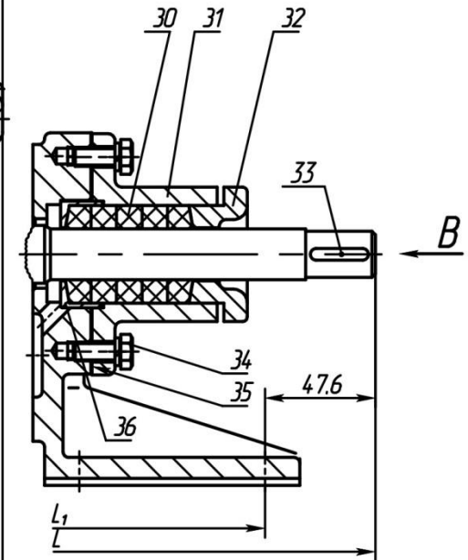
Рисунок А.2 (остальное см. рисунок А.1) Размеры в мм
