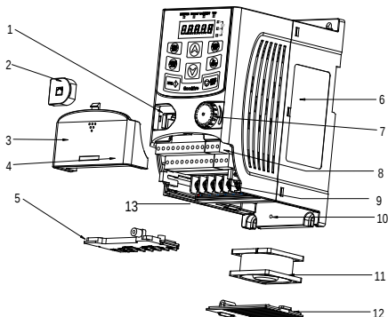
Рис. 2-3 Структурная схема ПЧ (3ф 380В, \leq 2.2 кВт)
