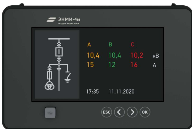
ЭНМИ-4м-220-4
