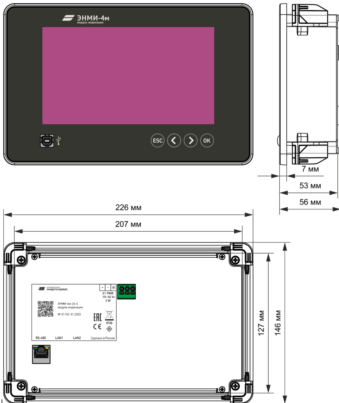
Рисунок 1.7. Габаритные размеры модуля ЭНМИ-Х-Х-4
