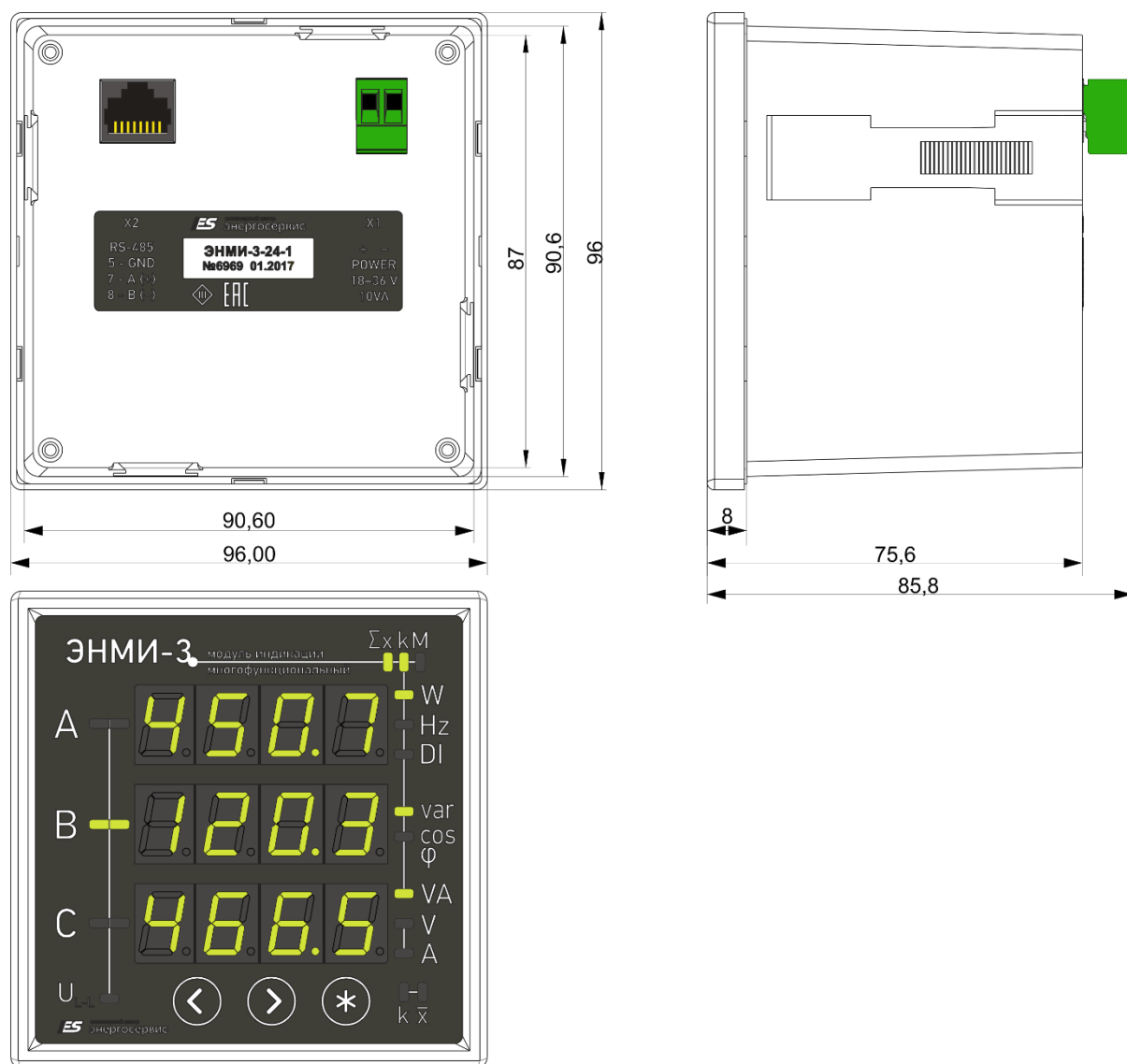
Рисунок 1.3. Габаритные размеры модификации ЭНМИ-Х-24-1
