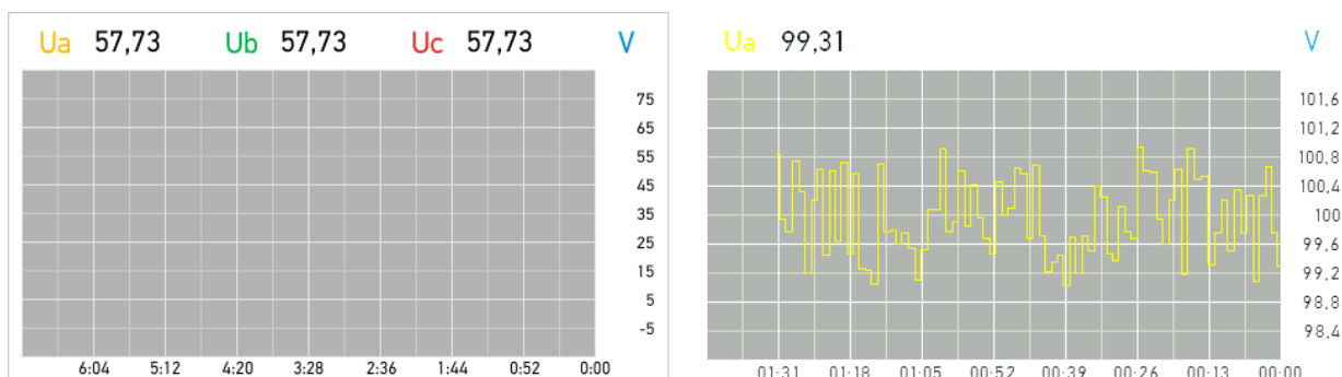
Рисунок 4.7. «Измерения» -> «Графики».
