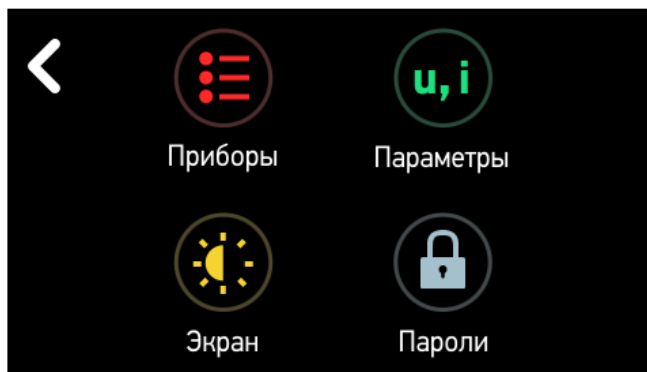
Рисунок 4.24. Меню «Настройки».
