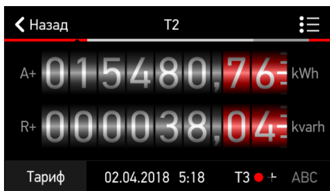
Рисунок 4.17. «Счетчик» -> «Табло».
