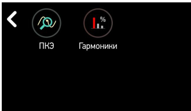
Рисунок 4.18. «ПКЭ».
