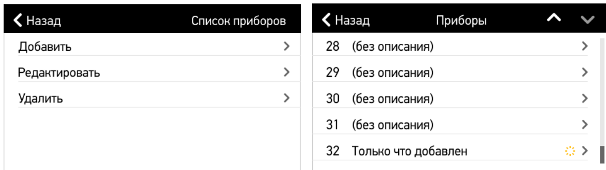
Рисунок 4.26. «Список приборов».
