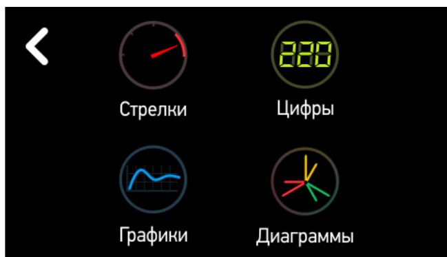
Рисунок 4.2. «Измерения».
