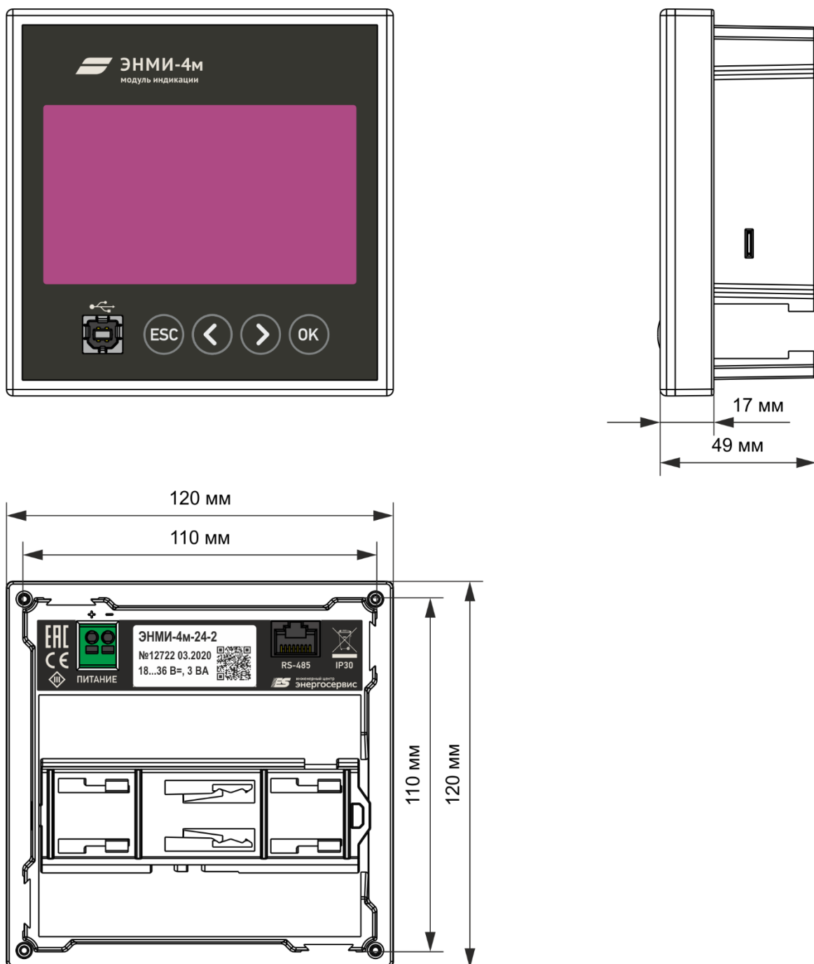
Рисунок 1.5. Габаритные размеры модуля ЭНМИ-Х-24-2Д
