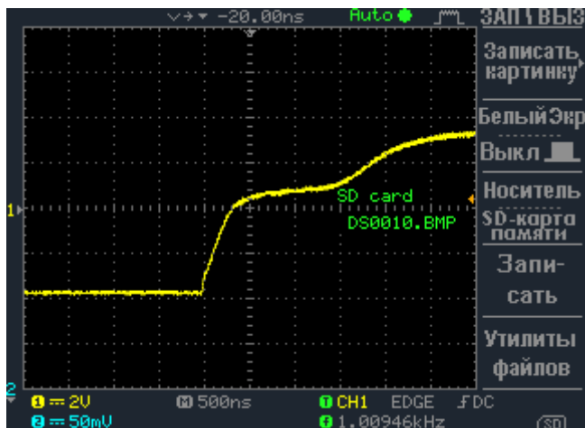
Рисунок 5.2. Линия с «оттяжками» 1 кОм. Видео: enip2.ru/files/rs485_02.zip
