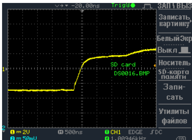
Рисунок 5.3. Линия, согласованная 1 кОм. Видео: enip2.ru/files/rs485_03.zip
