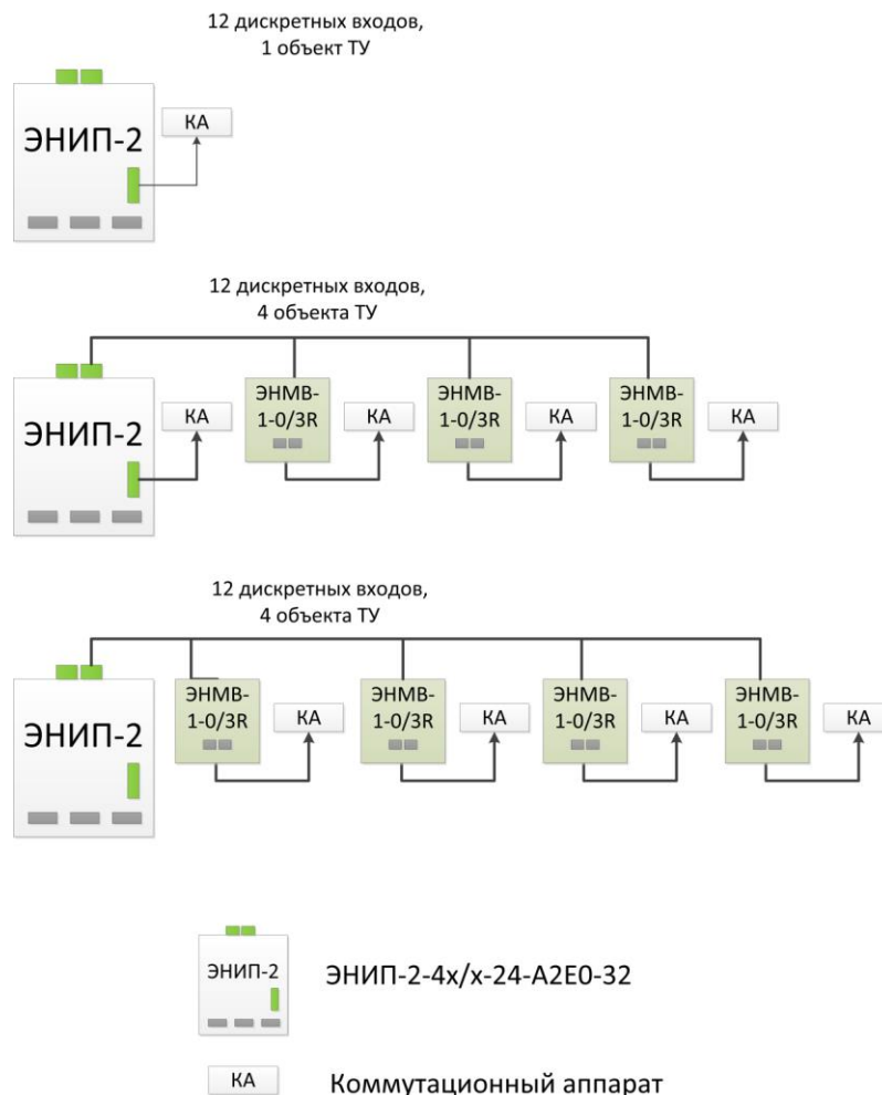
Рисунок 8.11. Схемы подключения ЭНИП-2-...-32 к внешним модулям
