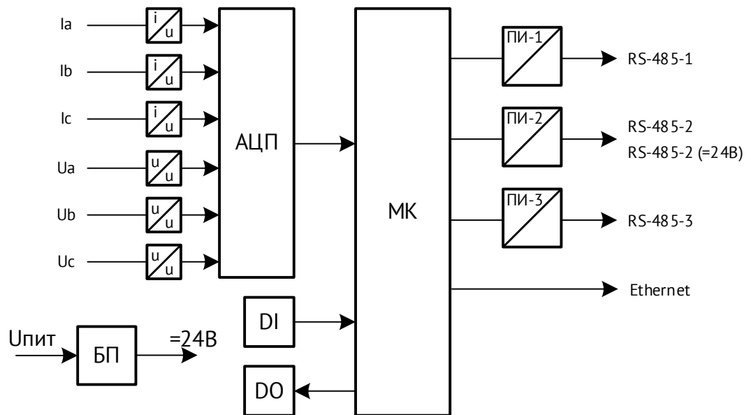
Рисунок 3.1. Структурная схема преобразователя ЭНИП-2-...-АЗЕ4-11
