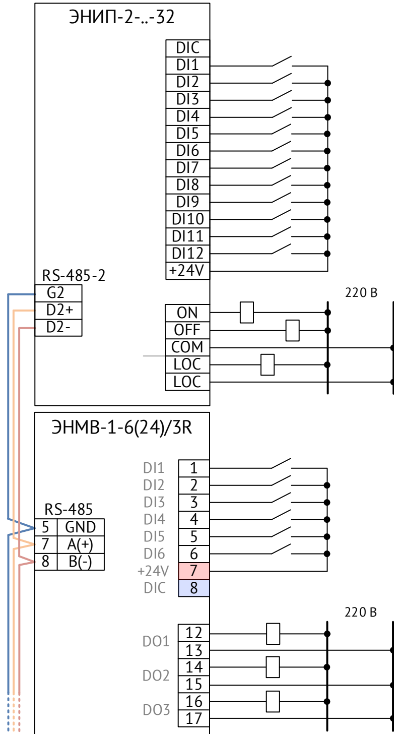
Рисунок 8.10. Схема подключения дискретных сигналов к ЭНИП-2-...-32. На примере вариант подключения дискретных входов с питанием от встроенного источника
