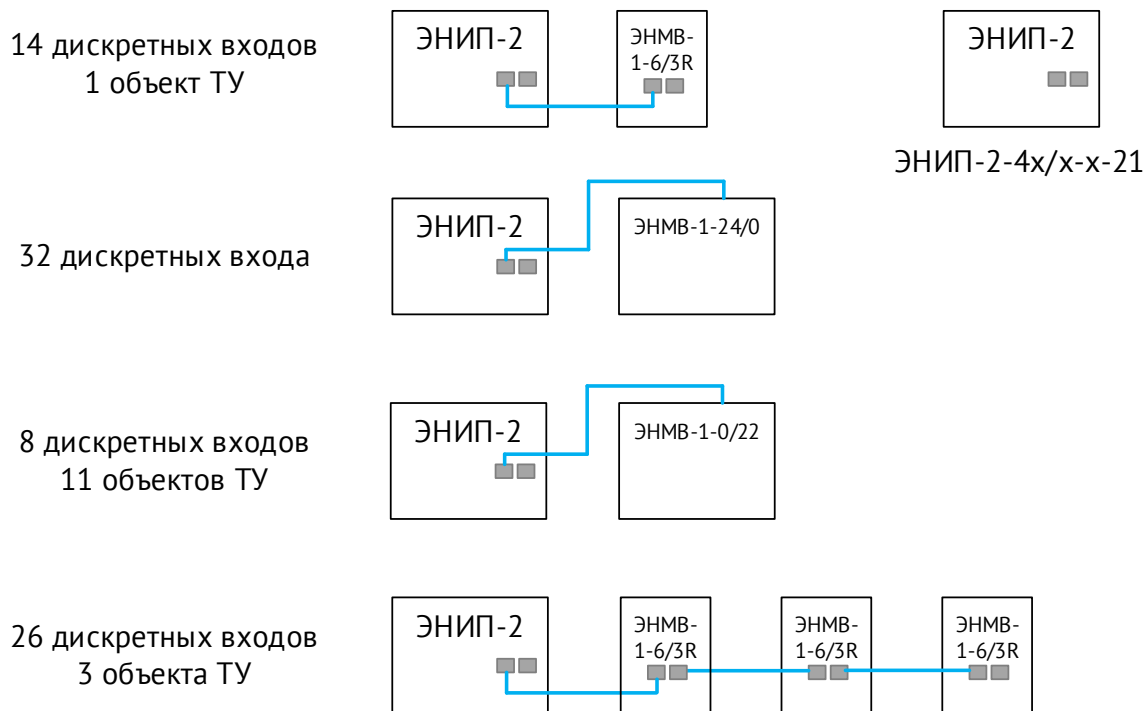
Рисунок 8.8. Примеры схем подключения ЭНИП-2-...-Х1 к внешним модулям
