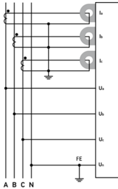
Рисунок А2.3. Схема подключения преобразователей ЭНИП-2-4Х/400-24-А2Е0-32 для трехфазной четырехпроводной сети 230 (400) В: 4LN3 или 4LL3 (ЭНИП-2 настроен на схему «4-проводная»)
