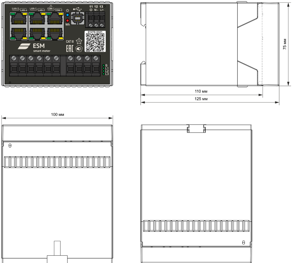
Рисунок 1.5. Габаритные размеры устройства ESM
