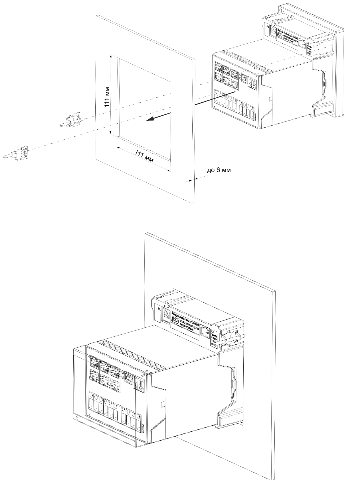
Рисунок 1.7. Схема установки устройства ESM с модулем индикации ЭНМИ-Х-24-2 в щит
