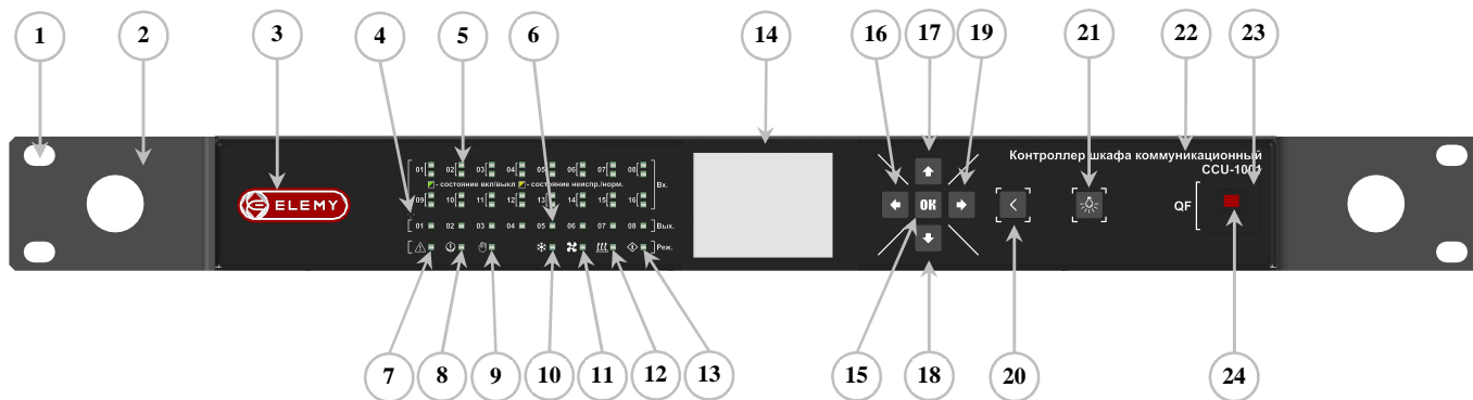
Рисунок 1 – Контроллер SCU-1001, передняя панель и кронштейны:
