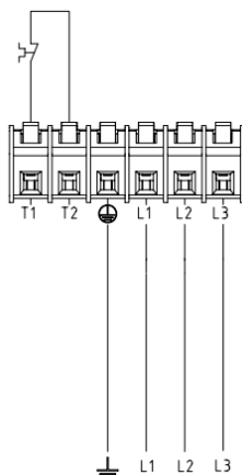
Рис. 10 Клеммы электрического подключения
