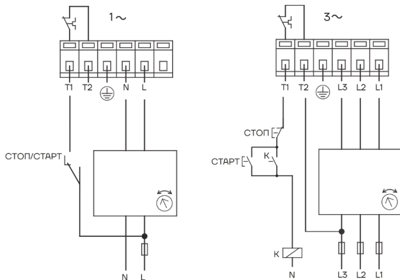
Рис. 15 Схема работы насоса, если защита обеспечивается с помощью реле перегрузки (защита электродвигателя по току), встроенный термодатчик используется
