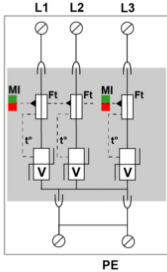
V: высокоэнергетический варистор Ft: тепловой предохранитель t ° : Система термического отключения MI: индикатор отключения
