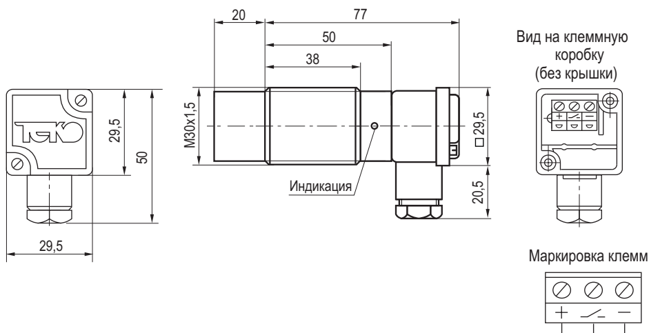
Габаритный чертеж
