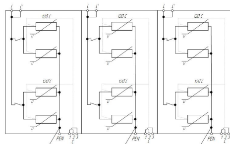
Схема электрическая принципиальная В-Т25 275 3+0 С
