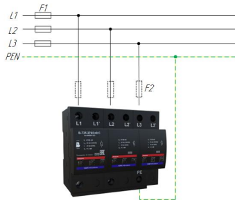
Схема подключения В-Т25 275 3+0 С для сетей с системой заземления типа TN-C
