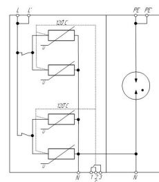
Схема электрическая принципиальная В-Т25 275/1+1 С
