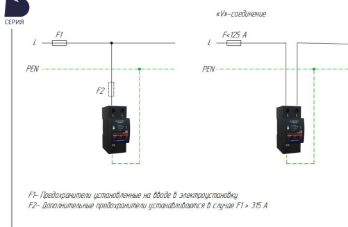
Схема подключения В-Т25 275 С для сетей с системой заземления типа TN-C
