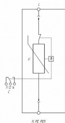
Схема электрическая принципиальная УЗМТ серии К2Р KB С
