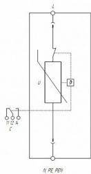
Схема электрическая принципиальная УЗМТ серии К2Р KB С
