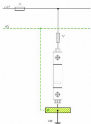
Схема подключения УЗМТ серии К2Р KB, К2Р KBP к сети с системой заземления типа TN-C
