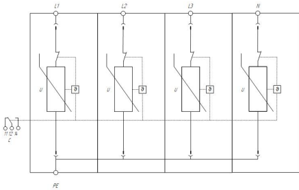
Схема электрическая принципиальная УЗМП серии К2Р КВ 4+0 С
