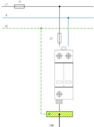
Схема подключения УЗМТ серии К2Р KB 240 С к сети с системой заземления типа TN-S
