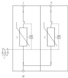
Схема электрическая принципиальная УЗМТ серии К2Р KB 240 С
