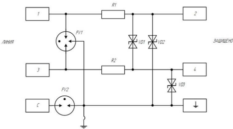
Схема электрическая принципиальная УЗМГ серии ГИС Л2
