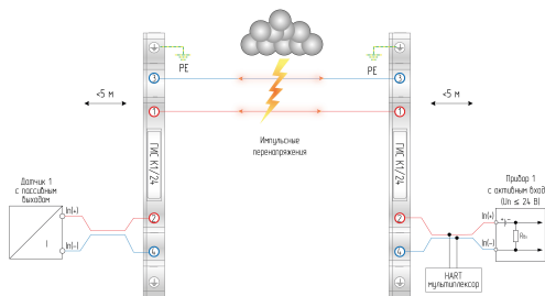
Пример схемы подключения ЗЭП серии ГИС К1/24 для линии интерфейса «Точка питания»
