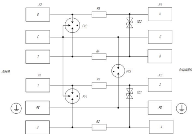
Схема электрическая принципиальная УЗО серии DTNVR 2F * / ** / *** G
