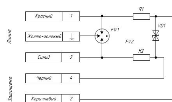
Схема электрическая принципиальная ГИК 110/2 Exd **
