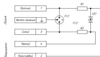
Схема электрическая принципиальная ГИК 30/• Exd **
