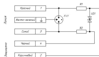
Схема электрическая принципиальная ГИК 24/2 Exd **
