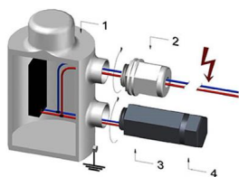
1- полевое устройство, 2- кабельный гермоввод, 3- УЗИП, 4- гайка-заглушка УЗИП
