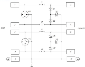
Схема электрическая принципиальная УЗМП серии РСТ 2
