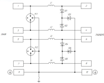
Схема электрическая принципиальная УЗМТ схем РСТ 2
