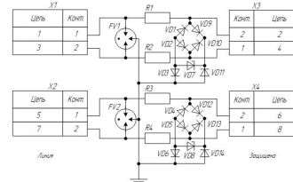
К2 КЛЮЧЕВОЙ КОМПОНЕНТ ЭНЕРГИЯ ВЕРНЫХ РЕШЕНИЙ | Схема электрическая принципиальная DT 2/4/5
