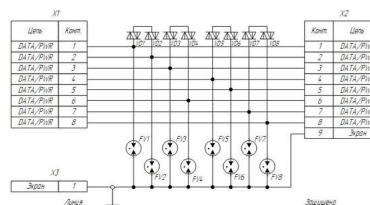
Схема электрическая принципиальная УЗИП ГИП 1.4/250М LSA/RJ
