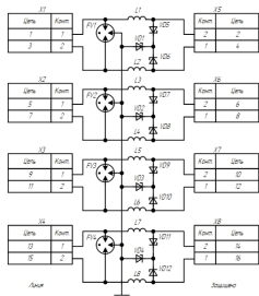
Схема электрическая принципиальная ГИП 4/350/5/1500
