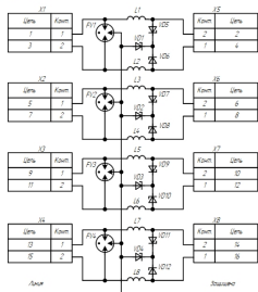
Схема электрическая принципиальная ГИП 4/220/5/1500
