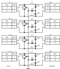
Схема электрическая принципиальная ГИП 4/48/5/1500
