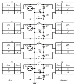
Схема электрическая принципиальная ГИП 4/24/5/1500
