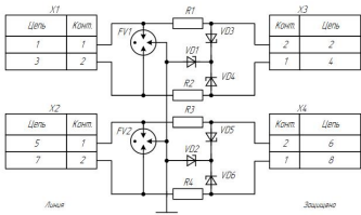
Схема электрическая принципиальная DT 2/Т/1500
