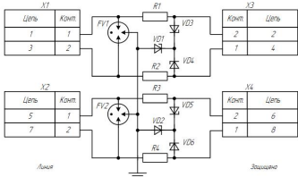
Схема электрическая принципиальная DT 2/110/1500
