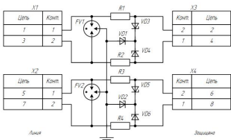
Схема электрическая принципиальная DT 2/30/1500
