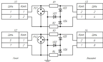
Схема электрическая принципиальная DT 2/**/1500
