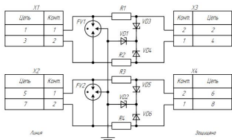
Схема электрическая принципиальная DT 2/6/1500
