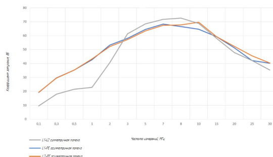
Характеристики запыления пачкоподводящего фильтра серии ГСФЗ 16 IT
