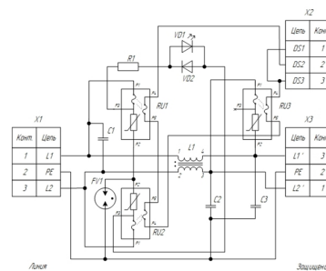
Схема электрических соединений ГСФЗ-48UC/16 IT
