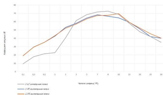
Характеристики затухания пассивного фильтра серии ГСФЗ 16 IT
