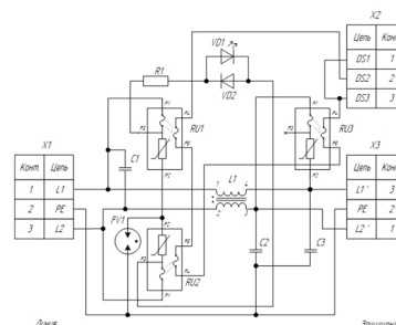
Схема электрических соединений ГСФЗ-230АС/16 IT
